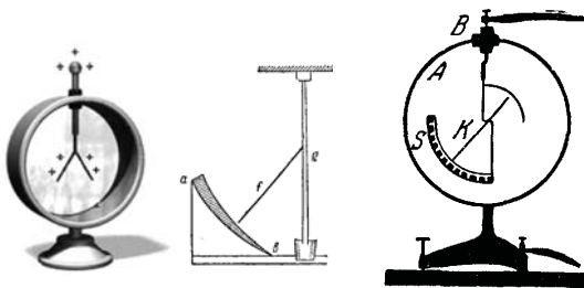
Электрометр Г.В.Рихмана (1745)
