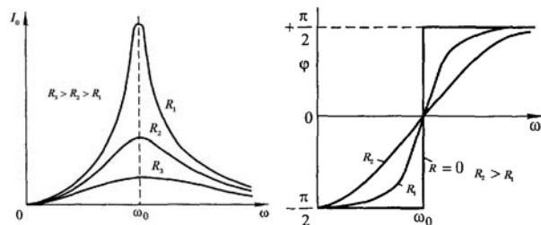
Резонансные кривые
