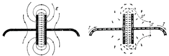
Электрическое поле в определенном момент времени. Величина поля E всюду уменьшается со временем. Ток проводимости (больше стрелки) и ток смещения (черные стрелки).
