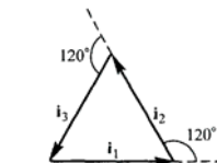
Векторная диаграмма токов в нулевом проводе. Симметричная нагрузка
