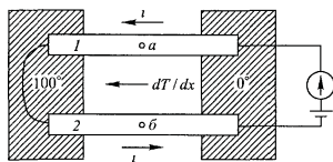
Рис. 344. Наблюдение эффекта Томсона
