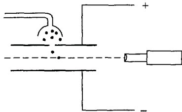
1.11. Схема опыта Милликана
