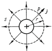
Электрическое поле в определенном момент времени. Величина поля E всюду уменьшается со временем. Ток проводимости (больше стрелки) и ток смещения (черные стрелки).
