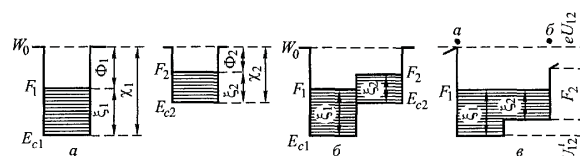
Рис. 339. Энергетическая диаграмма двух металлов: а — контакта нет; б — контакт есть, но нет равновесия; в — равновесие
