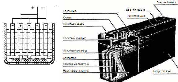
Рис. 3.2. Устройство VRLA-батарей Panasonic
